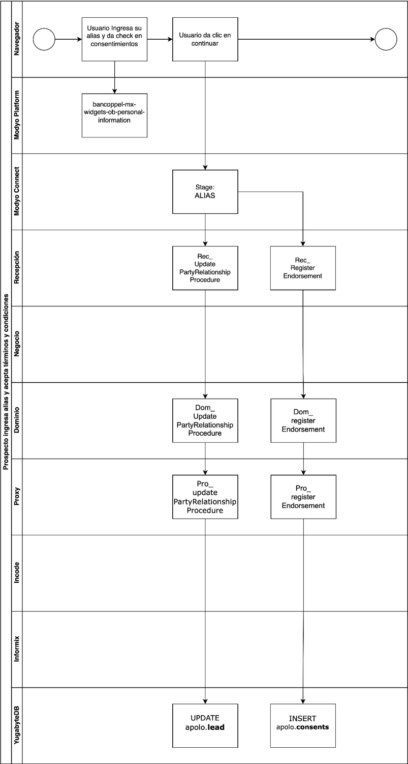
Diagrama de flujo de la arquitectura 2. TyC & Aviso de privacidad
