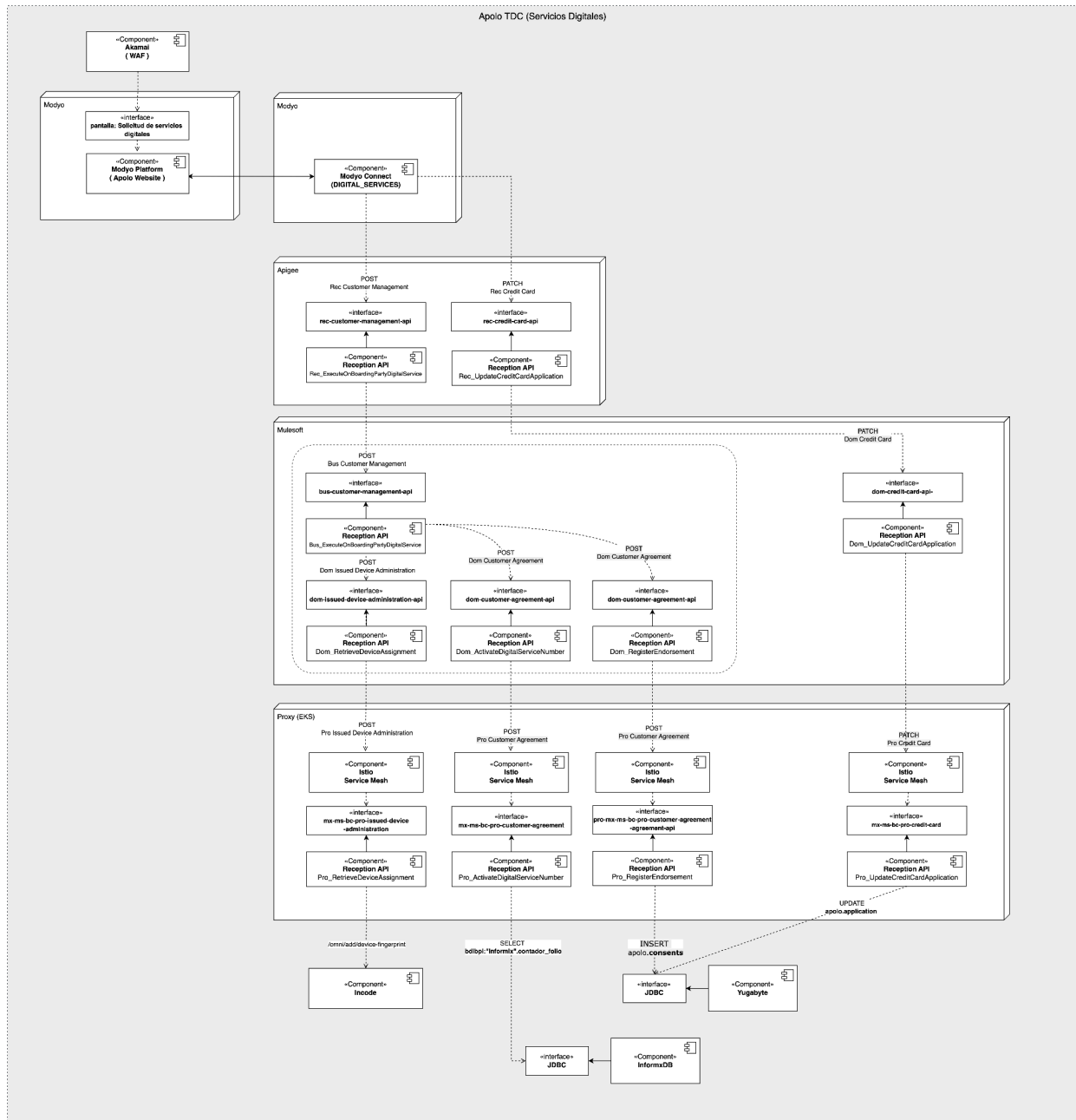
Diagrama de Interfaces - Servicios Digitales
